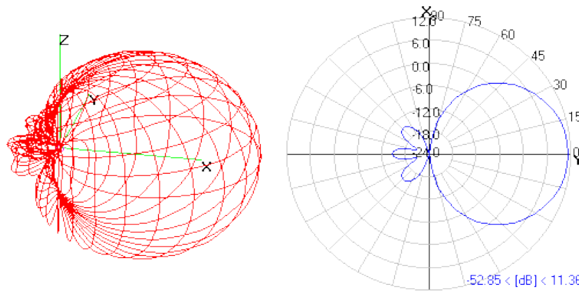
Antena direccional
